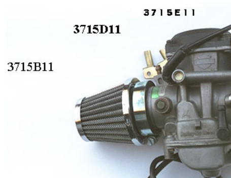
3715B11 Filtra aria a Cono da 40mm 3715D11 Filtra aria a Cono da 52mm 3715E11 Filtra aria Cono con attacco da 54mm. (04-82)
