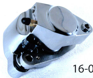
16-0714 Kit pinza anteriore sinistra per H-D dal 1984 fino al 1999 cromata.(14-08)
